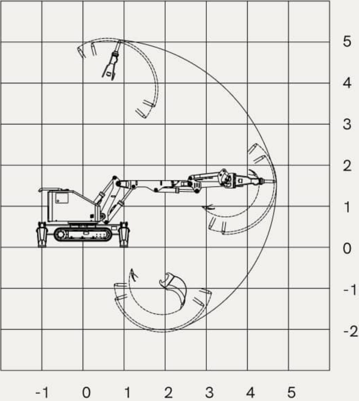
Рабочая зона стрелы
